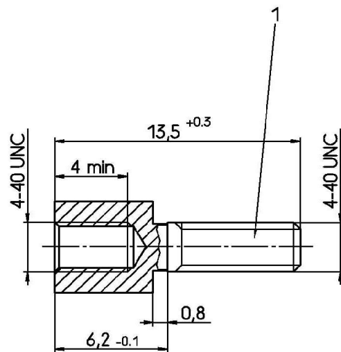
Sechskant SW 4,5
