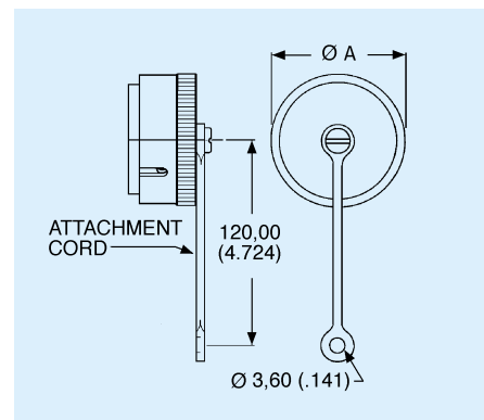
Receptacle Dust Cap
