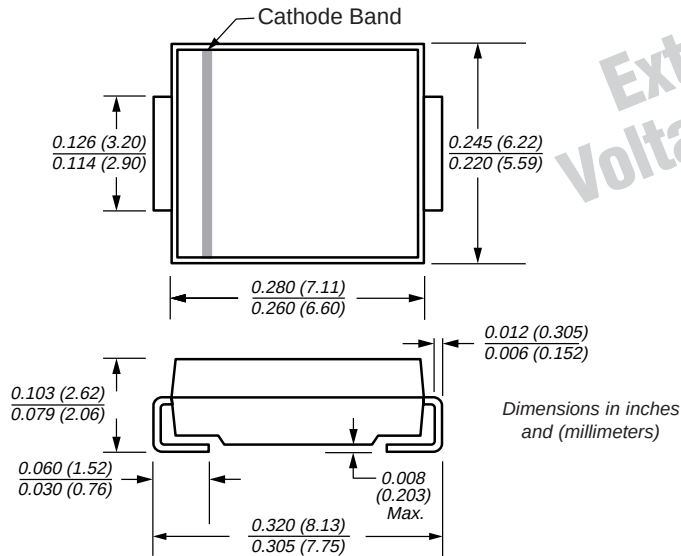
DO-214AB (SMC J-Bend)
