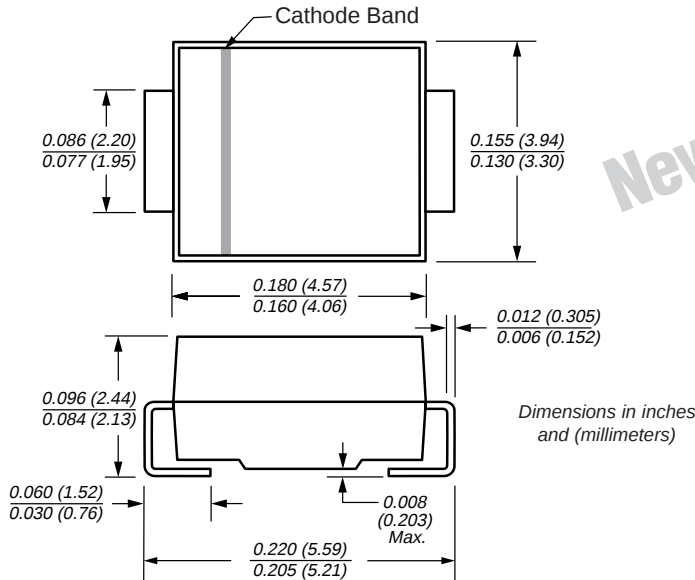
DO-214AA (SMBJ)
