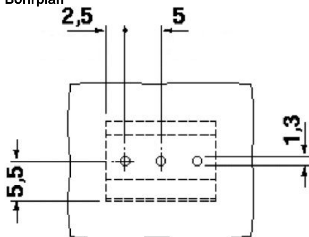
Maßzeichnung
