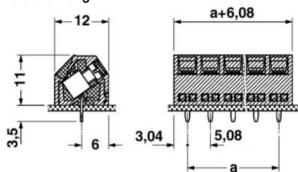
Maßzeichnung
