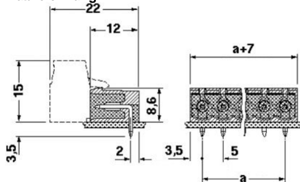
Maßzeichnung
