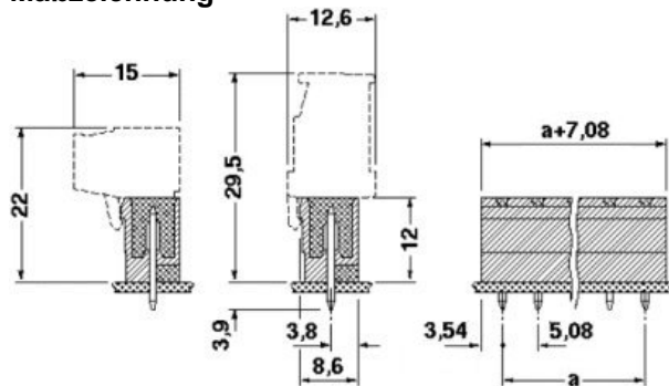
Maßzeichnung
