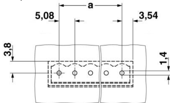
Maßzeichnung
