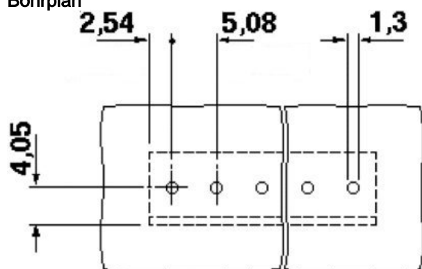
Maßzeichnung
