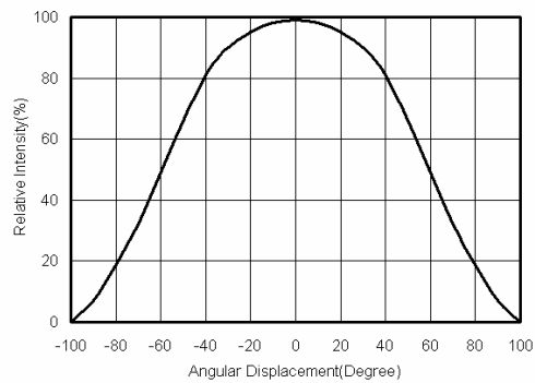
EDEI-1LA3 & EDEI-ALA3
