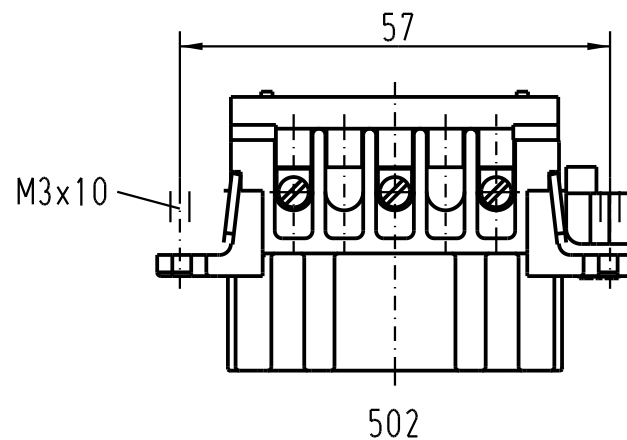
Kontaktanordnung (Ansicht Anschlussseite) contact arrangement (view from terminal side)
