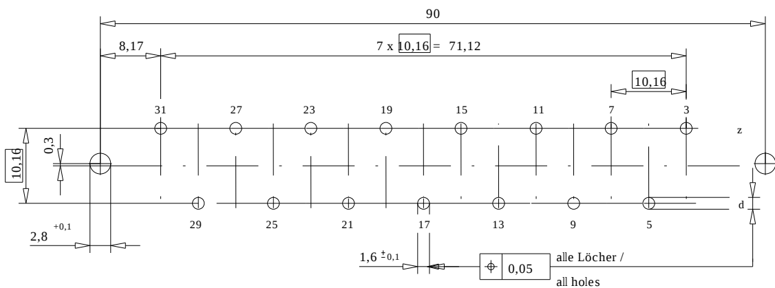
Leiterplatten-Lochbild / PCB drillhole pattern
