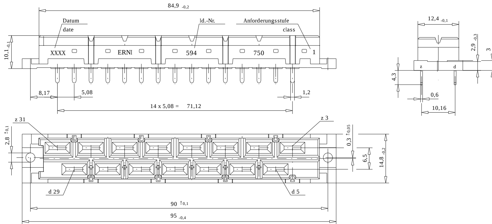
Bestückungsplan / contact layout
