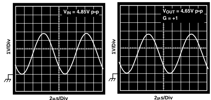
Input V_{IN}
