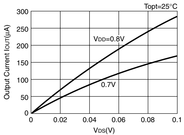
R3111x09xC
