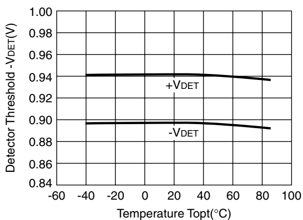
R3111x09xC
