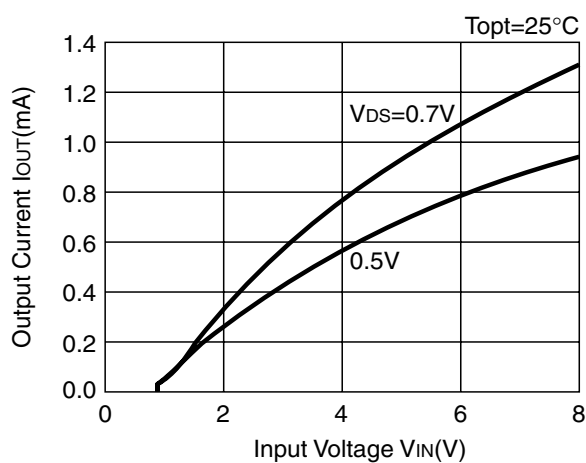
R3111x09xC
