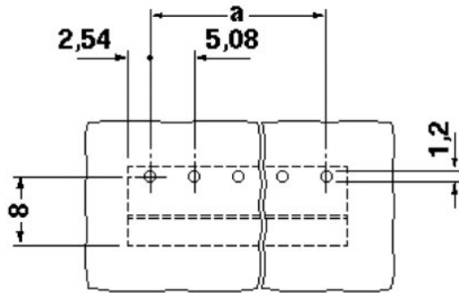
Bohrplan
