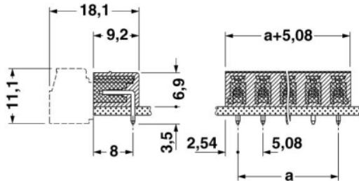
Maßzeichnung
