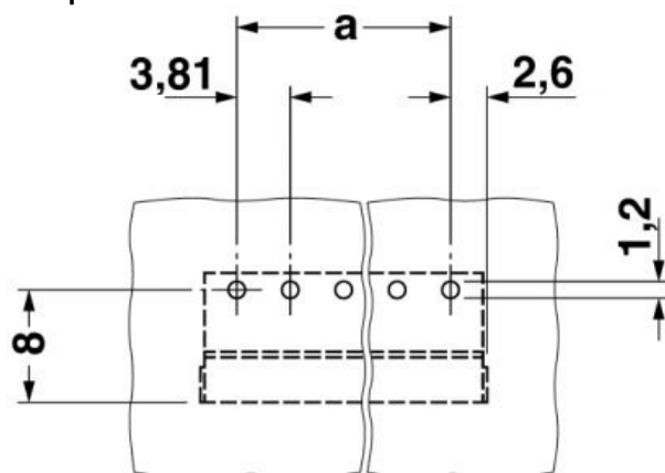
Maßzeichnung
