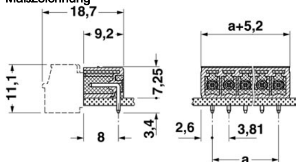
Maßzeichnung
