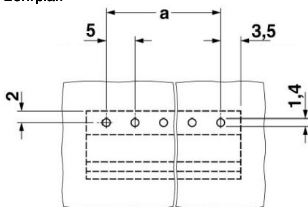
Maßzeichnung
