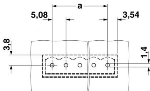
Bohrplan
