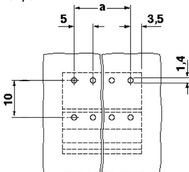
Maßzeichnung
