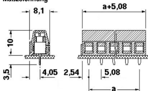
Maßzeichnung
