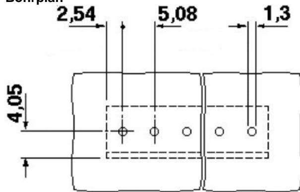
Maßzeichnung
