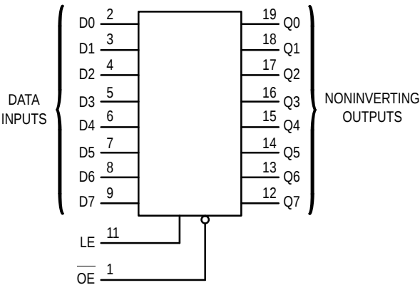
FUNCTION TABLE
