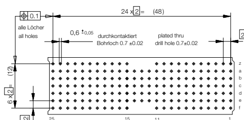
Lochbild fuer Leiterplatte (Bestueckungsseite)
