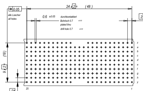
Lochbild fuer Leiterplatte (Bestückungsselle)
