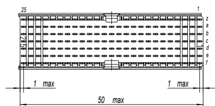
Lochbild fuer Leiterplatte (Bestueckungsseite)
