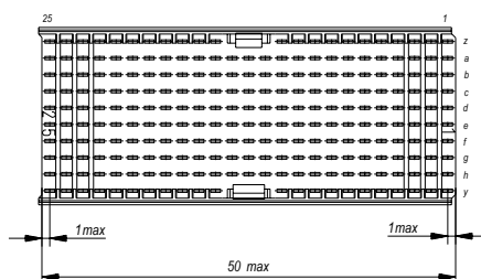
Lochbild fuer Leiterplatte (Bestückungsselle)
