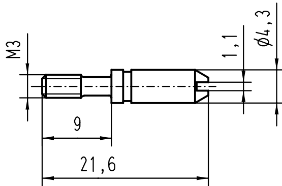
Führungsstift / guide pin
