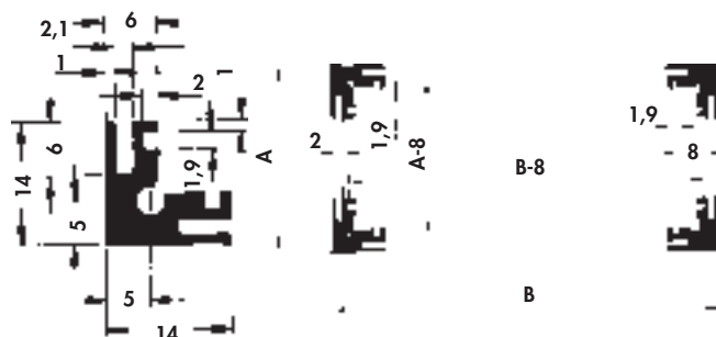
Eckprofil / Edge profile / Profilé d'angle GB 1
