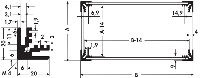
Eckprofil / Edge profile / Profilé d'angle GB 66
