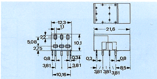
Steckverbinder DIN 41649
