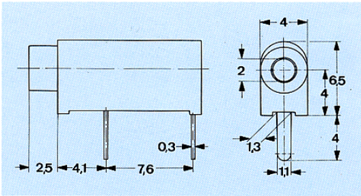
Steckverbinder DIN 41649
