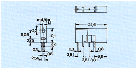
4-polige Prüf- und Schaltbuchse
