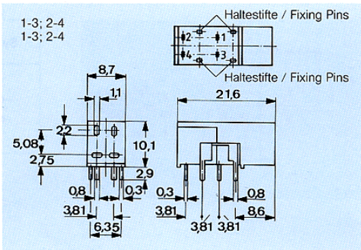
4-polige Prüf- und Schaltbuchse
